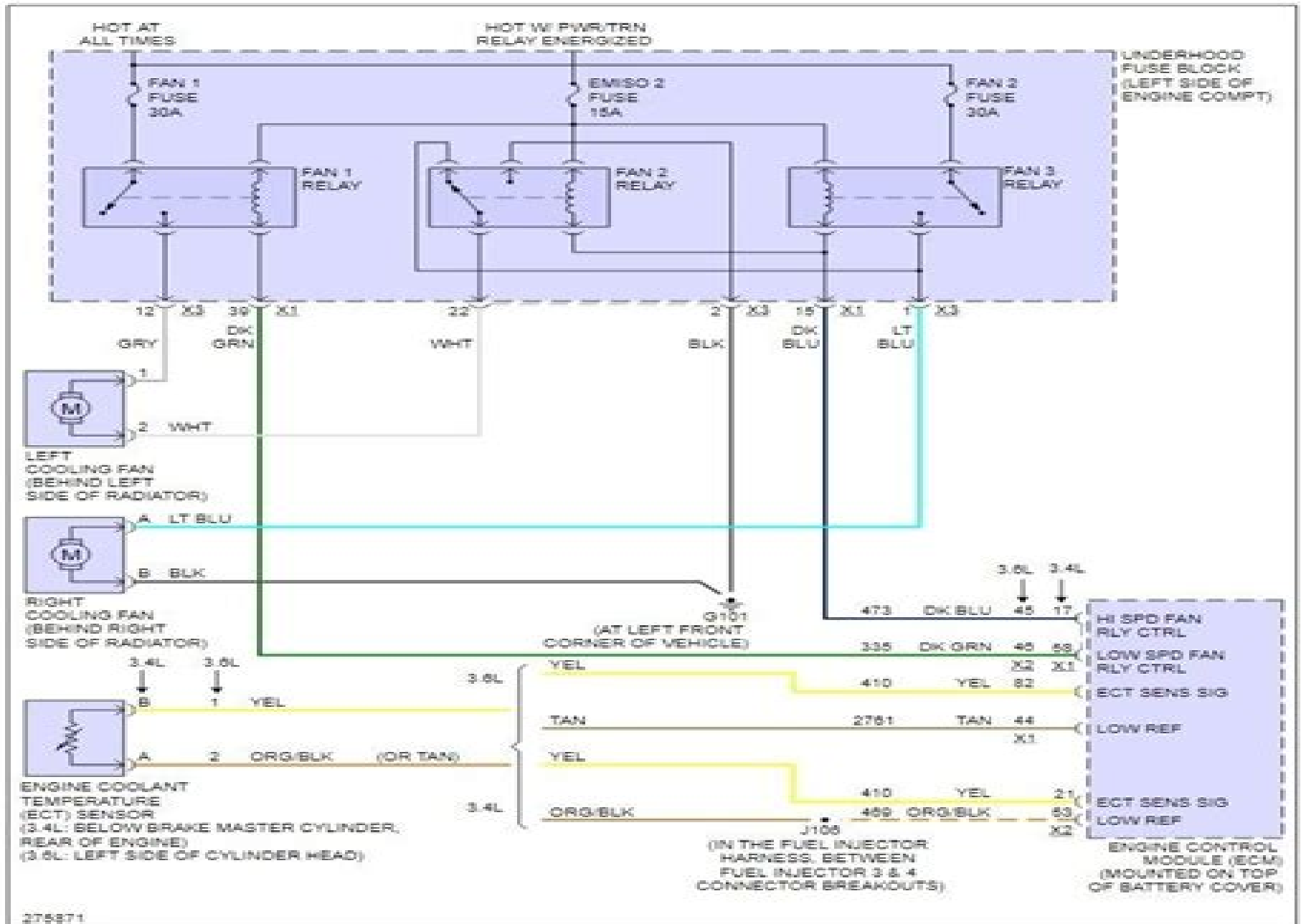
Fig 1: Cooling Fan Circuit
