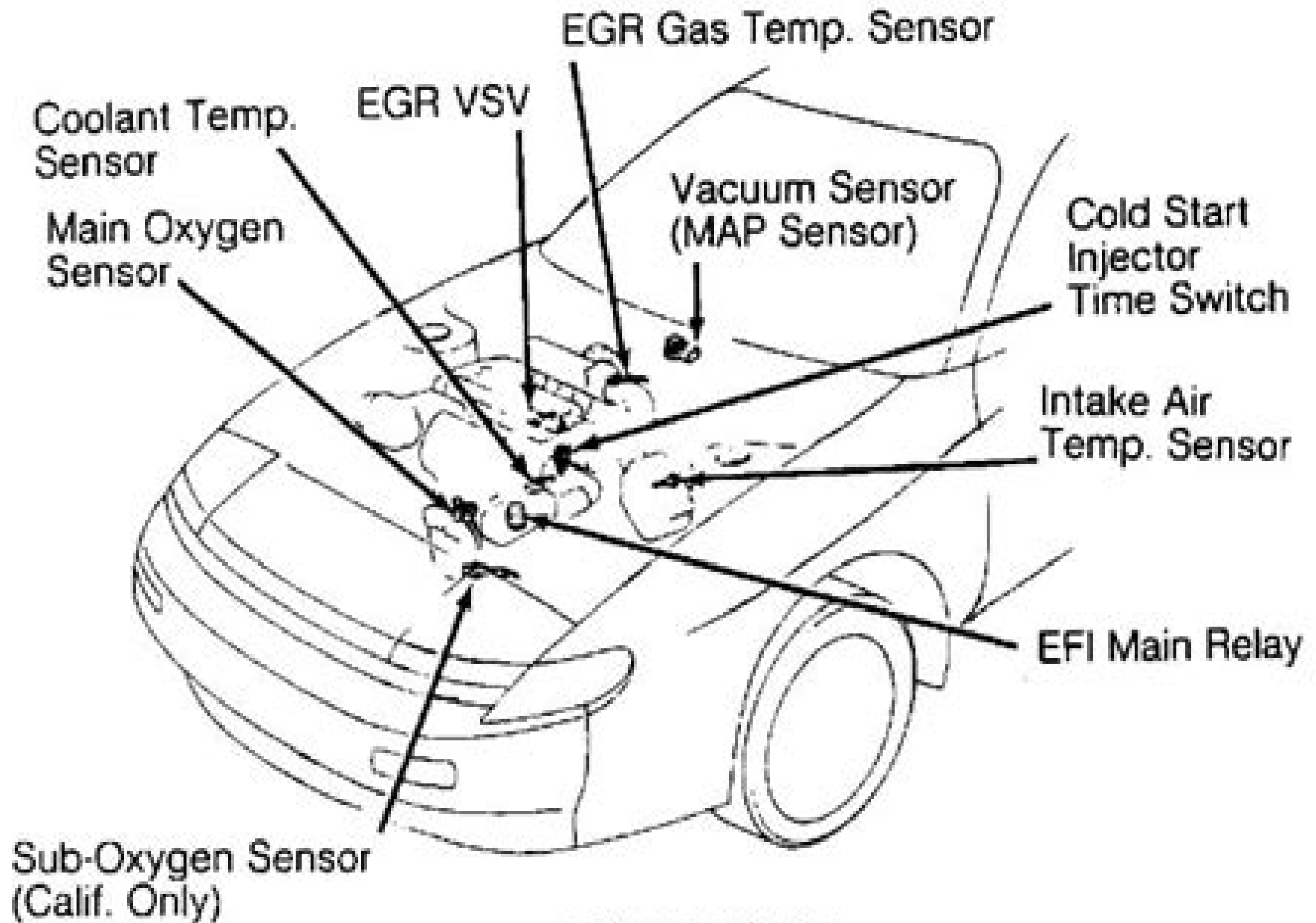
CELICA (5S-FE)
